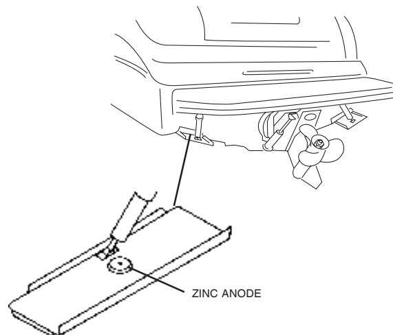
ZINC ANODE (FIG. 6.7.1)
