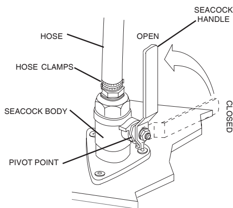
SEACOCK (FIG. 8.6.1)
